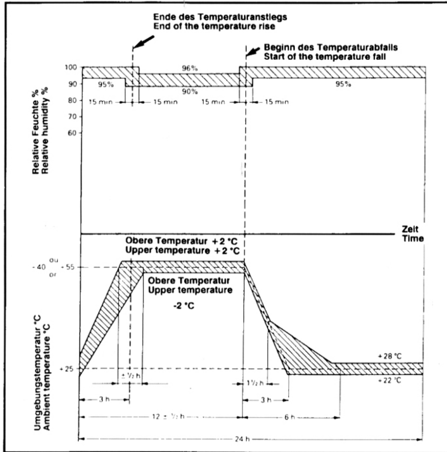
DIN-IEC 68, Teil 2-30 Test Db, Variante 1
