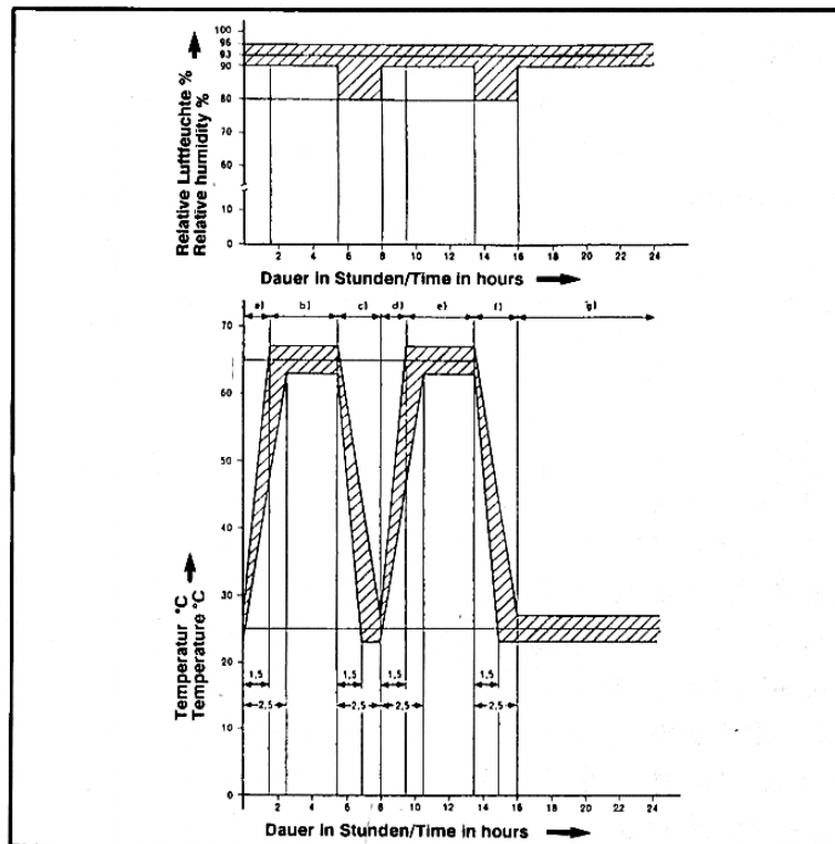
DIN-IEC 68, Teil 2-38 Test Z/AD
